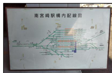
南宮崎駅構内配線図
