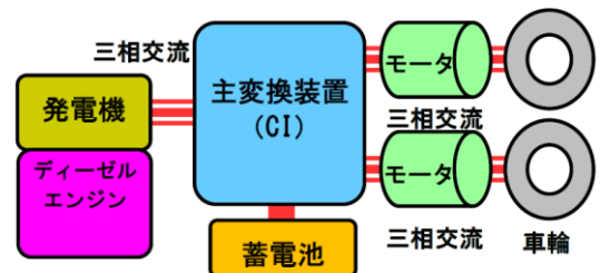
○蓄電池搭載型ディーゼルエレクトリック車両
